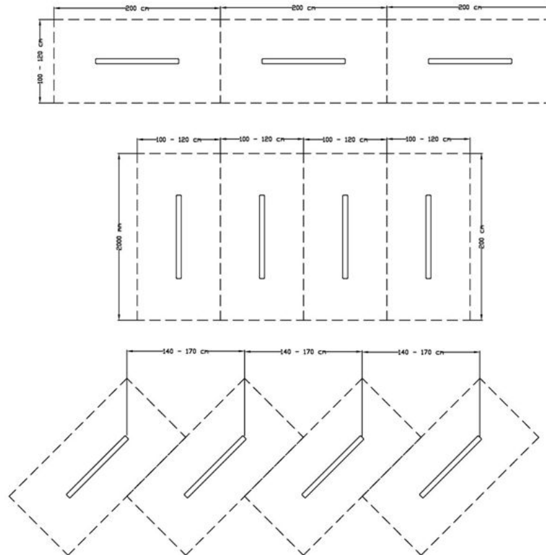
Rysunek 4.2 Schematy usytuowania miejsc parkingowych
