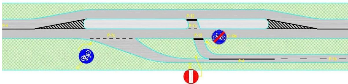
Rysunek 3.3 Zakucie dwukierunkowej drogi dla rowerów z wprowadzeniem ruchu rowerów w jezdni
