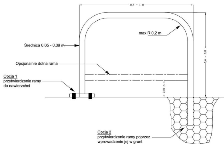
Rysunek 4.1 Schemat stojaka rowerowego w kształcie odwróconej litery „U” ród: opracowanie własne na podstawie Standardów projektowych i wykonawczych dla systemu rowerowego w m.st. Warszawie
