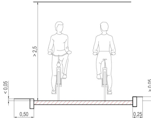
Rysunek 3.1 Wymiary skrajni dla rowerów [m]
