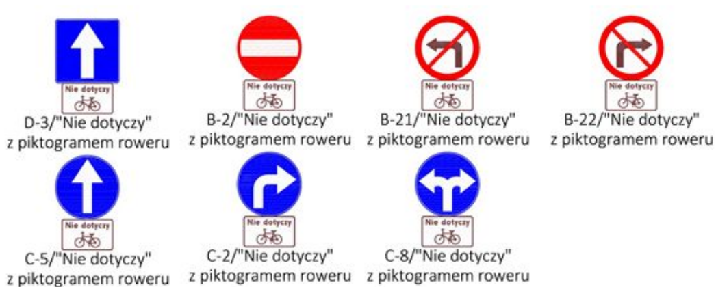
Rysunek 3.5 Zestaw znaków z dopuszczeniem ruchu rowerowego oznaczonym tabliczką „Nie dotyczy” z symbolem roweru
