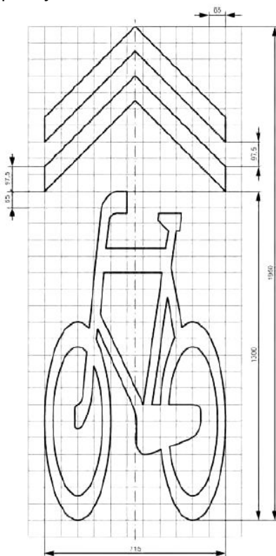
Rysunek 3.2 Znak P-27
