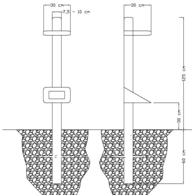
Rysunek 4.3 Schemat podpórki rowerowej
